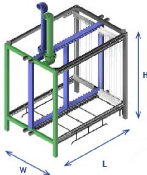
50 Module Skid
