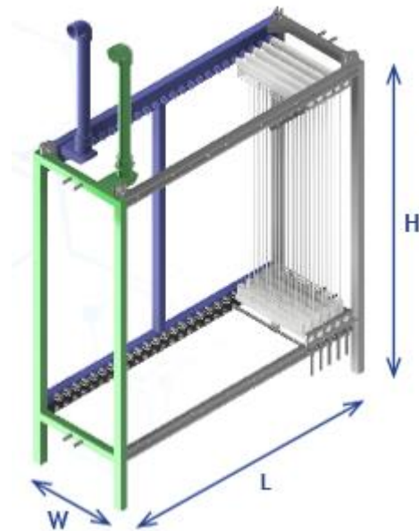
25 Module Skid
